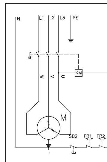
Schéma zapojení 400V~50Hz
