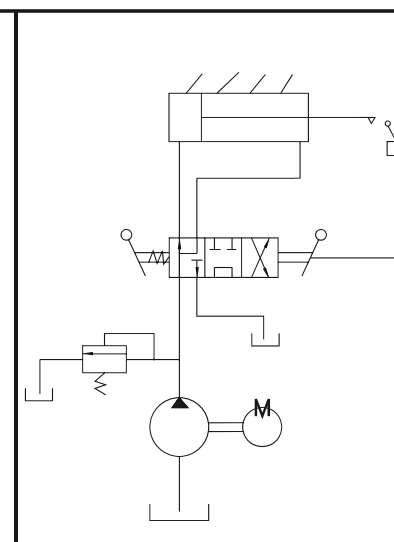
Hydraulické schéma
